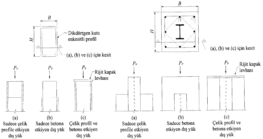
Şekil 12.8 – Kompozit kolonda dış yük etkisi
