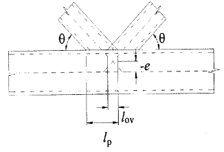
(b) Bindirmeli K-birleşimi
