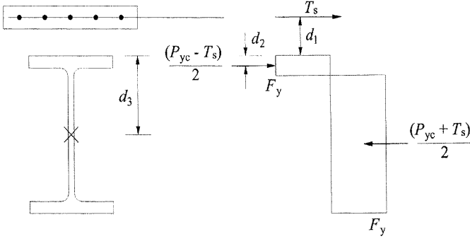
Şekil 12.3 – Kompozit kirişte negatif eğilme momenti için genel plastik gerilme yayılımı
