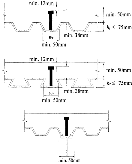
Şekil 12.4 – Şekil verilmiş çelik sac için konstrüktif esaslar
