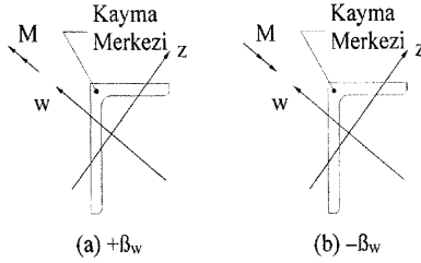
Şekil 9.2 – Eğilme momenti etkisindeki farklı kollu korniyerler için \beta_w işareti tanımı
