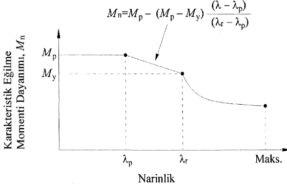
Şekil 12.5- Beton dolgulu kompozit kirişlerde karakteristik eğilme momenti dayanımı
