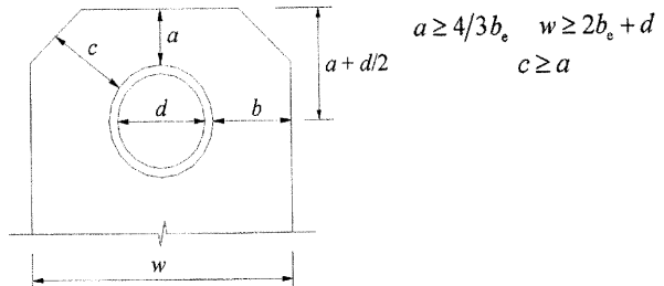
Şekil 13.11 – Çekme elemanlarının mil birleşimleri için boyutlar
