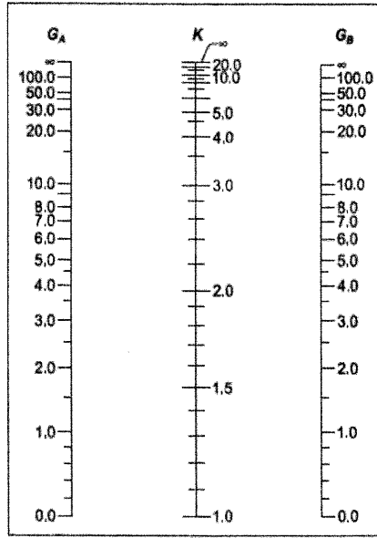
Şekil 6.2 – Yanal yerdeğiştirmesi önlenmemiş sistemlerde burkulma boyu katsayısı, K
