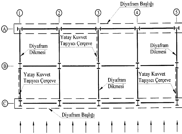
Şekil Ek 3.1 – Tipik yük aktarma elemanları (diyafram dikmeleri) ve diyafram başlıkları
