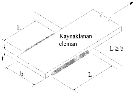
Şekil 13.3 – Sadece boyuna kaynak uygulanan uç birleşimi
