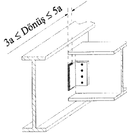
Şekil 13.7 – Kiriş ucu ile birleşim elemanı arasındaki dönme uyumunun sağlanabilmesi için kaynak uygulaması
